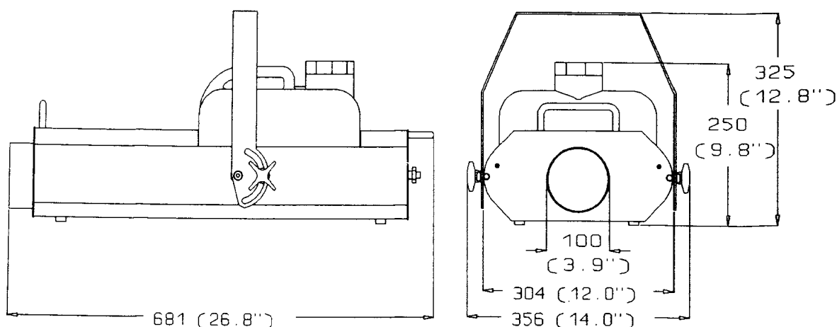
Abb.1: Abmessungen in mm
